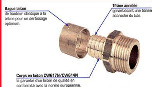
RACCORDS A SERTIR PAR GLISSEMENT
